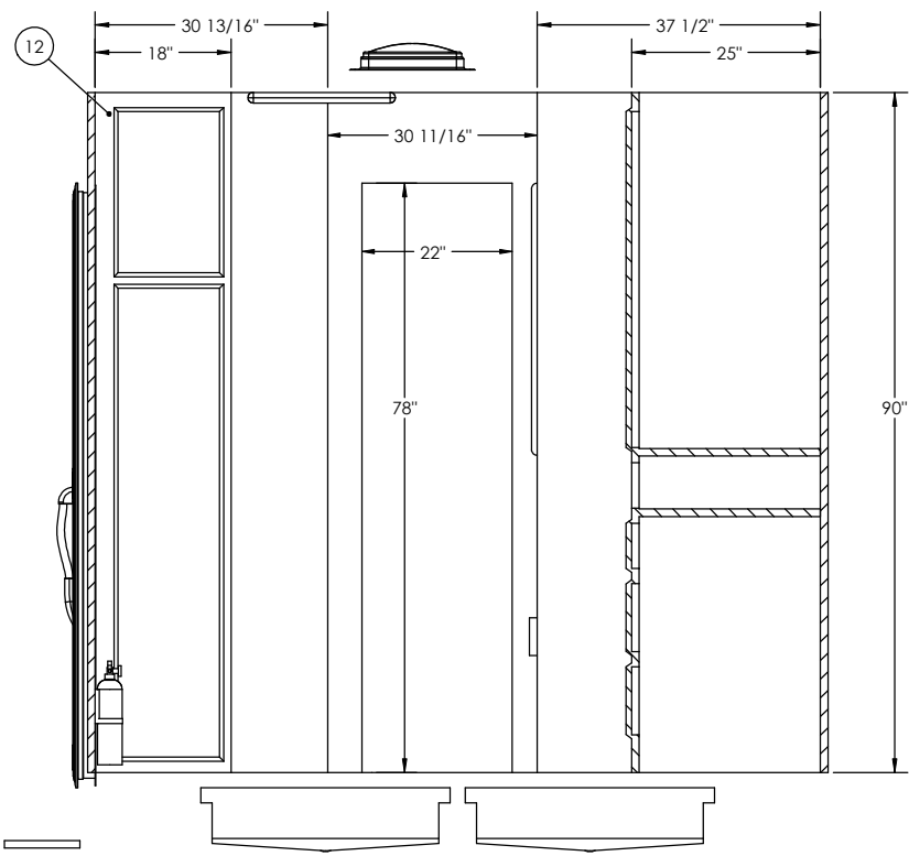
SECTION D-D
